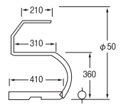
③ SW18-8 S型 3段ピュアー ケーキスタンド [NWCS-03] 13-0795-0301 ¥227,500 サイズ:510×φ410×H600
