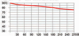
温度変化グラフ【保熱】
