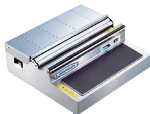
⑤ピオニー 18-8 ポリパッカー PE-405B (DX)
