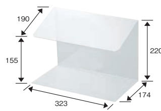
⑦ セーフティバリア ミニ
