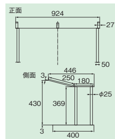
② EBM フードガード 片面
