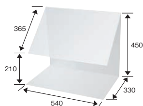
⑥ セーフティバリア
