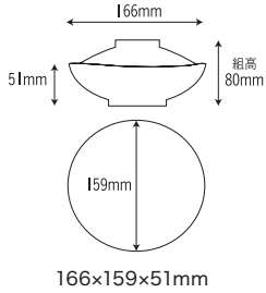
2529-OT [帯十草] 容量: 480ml 重量: 148g 価格: 身 ¥1,260 蓋 ¥1,140 → p 79
