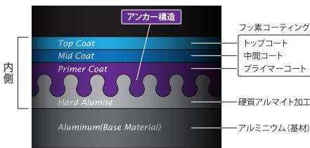
フッ素コーティング フライパン断面図
