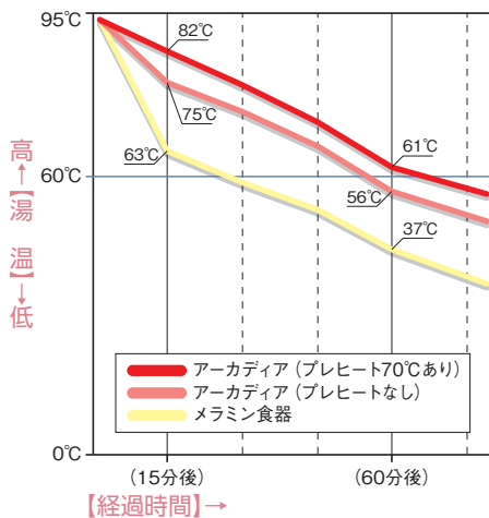
保温データ 条件：汁椀（お湯95℃）180ml 室温23℃
